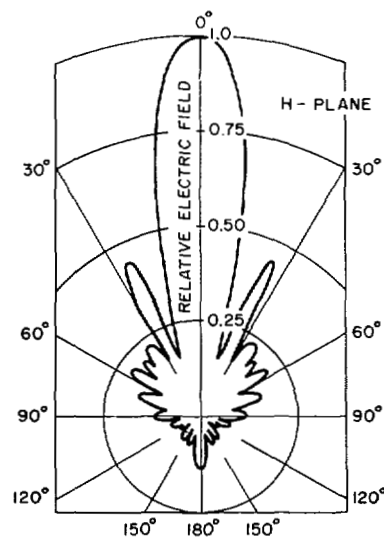
Fig. 8. H -plane pattern for array of Fig. 7.
